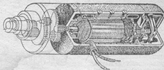
Tak wygląda mikrosilniczek w przekroju. Ten miniaturowy Herkules rozwija moc 3 KM przy 120 000 obr./min. Po lewej stronie widać przekładnię zębatą.
