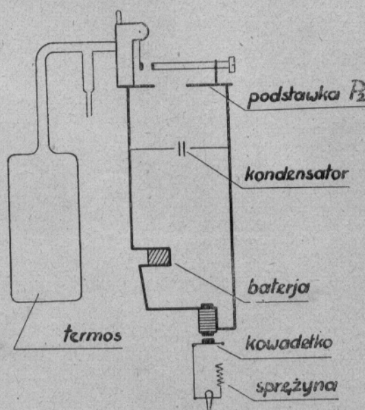
Schematy urządzenia wario-sterowania
