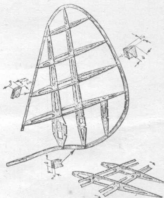
Montaż statecznika pionowego
