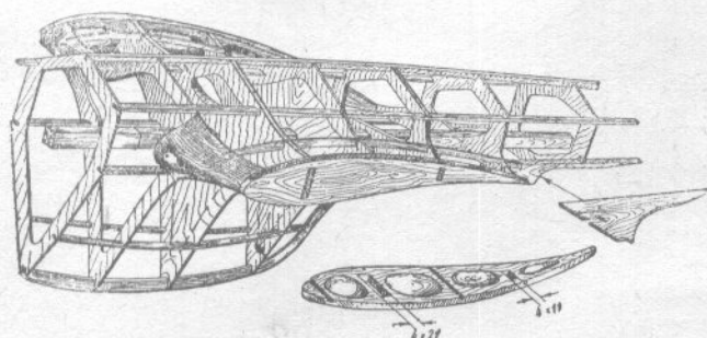
Przykładowe łączenie skrzydeł.
