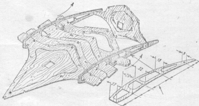
Montaż wręg przyskrzydłowych
