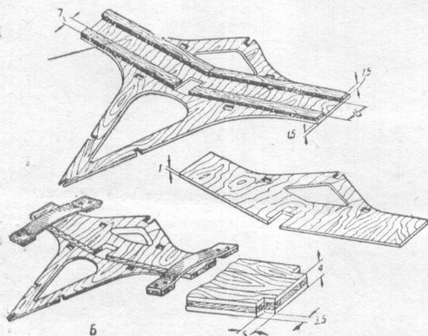
Wręga środkowa z łączem
