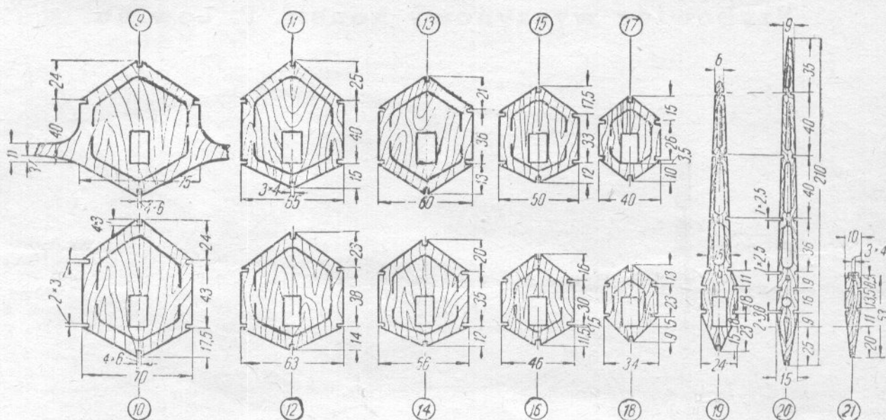
Wręgi kadłuba i statecznika
