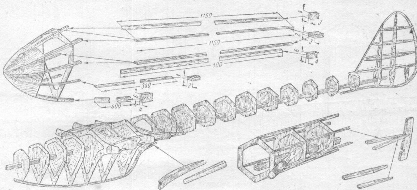
Budowa kadłuba i montaż wręg na beleczce.
