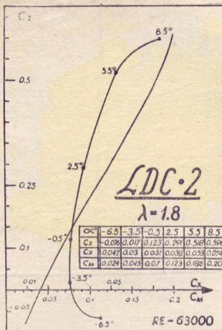
Biegunowa profilu laminarnego LDC-2
