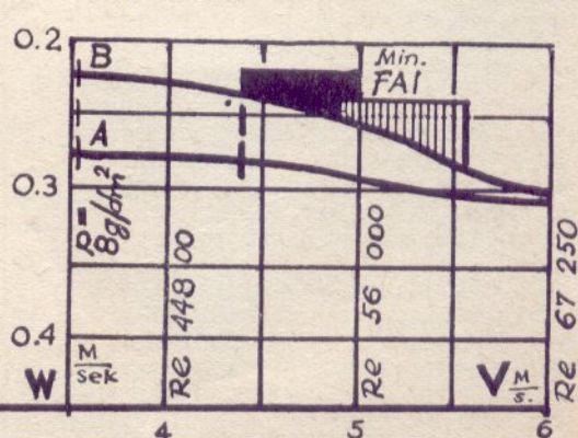
Wykres prędkości lotu V i opadania W.
