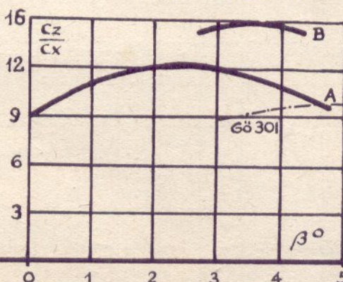
Krzywa doskonałości modelu
