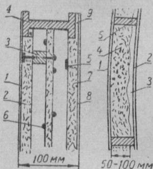
Rys. 1. Przekrój ściany w kabine nowoczesnego samolotu. 1 — ścianka zewnętrzna, 2 — korek (lub futro, wata, bawełna), 3 — żeberko, 4 — ściągacz, 5 — pasek skórzany, utrzymujący futro, 6 — linki sznurowe, 7 — futro, 8 — ścianka wewnętrzna, 9 — żeberka drewniane.
