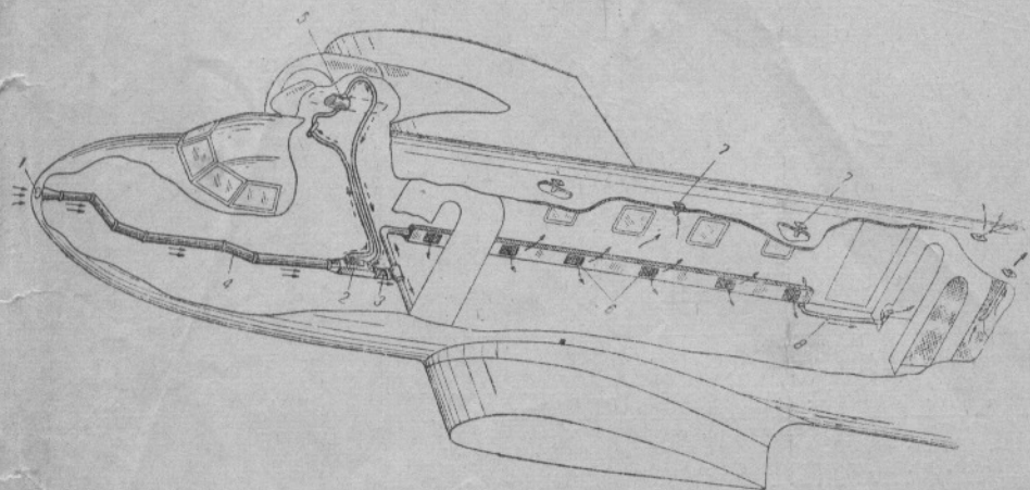
Rys. 6. Poglądowy schemat ogrzewania i wentylacji kabiny. 1 — otwór, przez który wlatuje powietrze do instalacji wentylacyjnej, 2 — podgrzewanie powietrza, 3 — filtr, 4 — przewód, 5 — zbiornik wody, ogrzewany gazami spalinowymi, uchodzącymi z silnika, 6 — wyloty wentylatorów, doprowadzające świeże powietrze do kabiny (mogą one być umieszczone w różnych miejscach kabiny), 7 — wylot zużytego powietrza odbywa się przy pomocy specjalnych zaworów, 8 — przewód doprowadzający powietrze do baru i pomieszczenia dla obsługi pokładowej.
