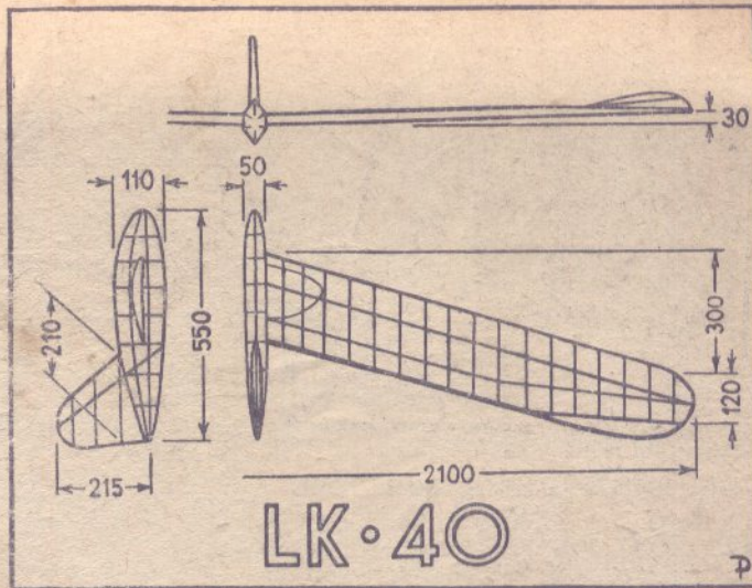
Szybowiec bezogonowy konstrukcji Lecha Komudy z Warszawy.
