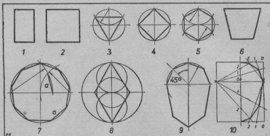
Wykreślanie różnych przekrojów kadłuba
