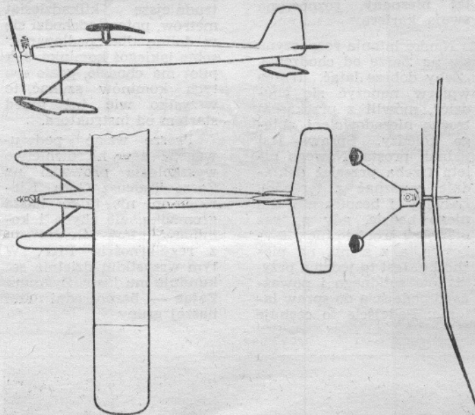
Model wodnoplata Wasilczenki (ZSRR)
