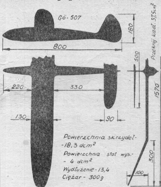
Szybowiec „Rekin” konstr. Pawła Elszteina. Plan tego modelu w skali 1:1 był wydany w 1947 roku przez redakcję SLM-U
