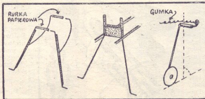
Rys. 3. Podwozie.
