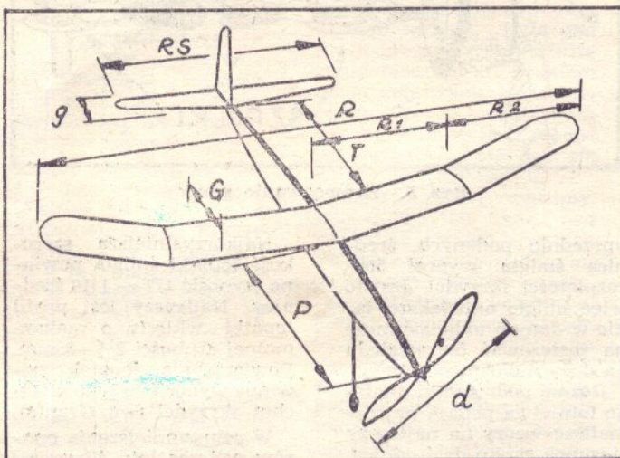
Rys. 1. Proporcje modelu rekordowego.
