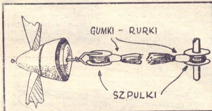
Rys. 5. Zamocowanie gumy
