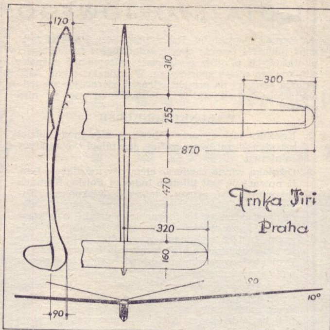
Szybowiec konstrukcji Ji-ri Trnka — Praha.
