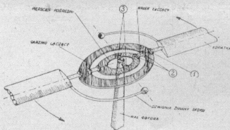
Rys. 3. Schemat głowicy przegubowej
