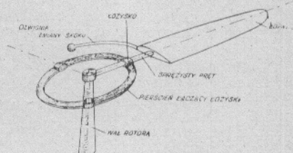
Rys. 4. Inny sposób polega na tym, że łopatki zakończone są sprężystym prętem
