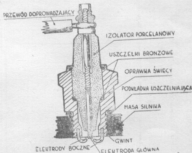
Rys. 12. Przekrój świecy
