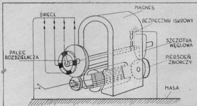
Rys. 8 — Ogólny schematyczny widok iskrownika
