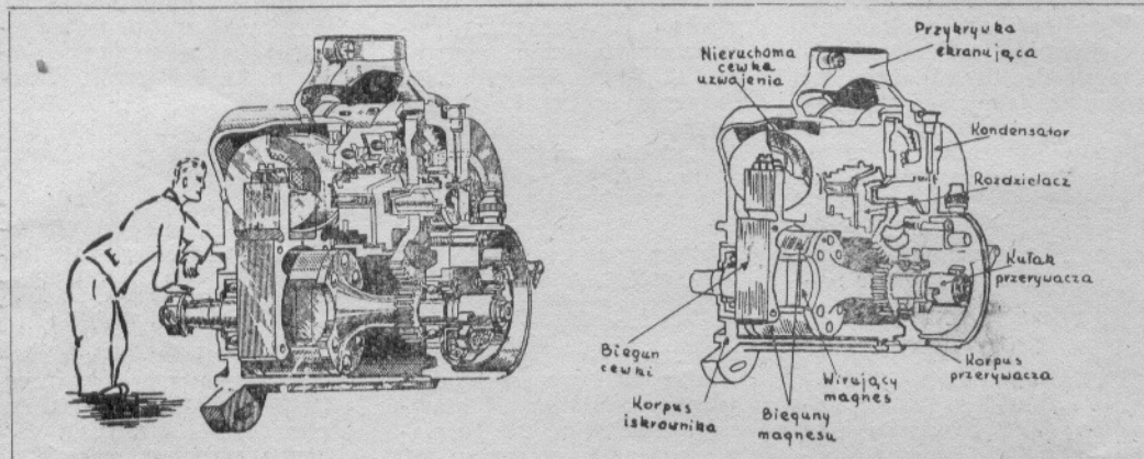
Rys. 9 — Przekrój iskrownika indukcyjnego
