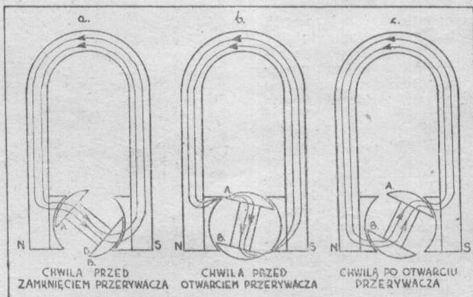
Rys. 7 — Schemat obiegu prądu w iskrowniku
