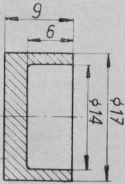
Tłok kompresyjny mat. dural, \phi 20 \times 30 ,
