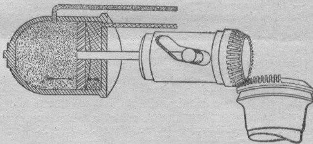
Rys. 16. Działanie napędu hydraulicznego radzieckiego śmigła AW. Zasada ta sama, co na rysunku dolnym
