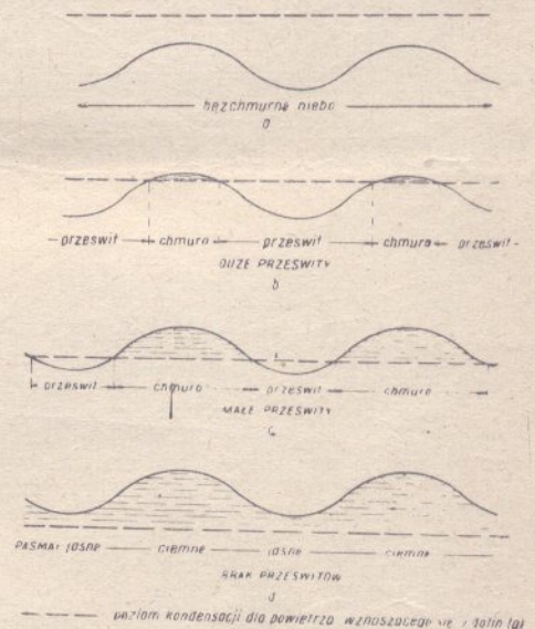
Rys. 4. Poziom kondensacji a uwidocznienie ruchów falowych
