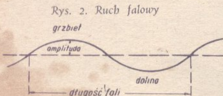
Rys. 2. Ruch falowy
