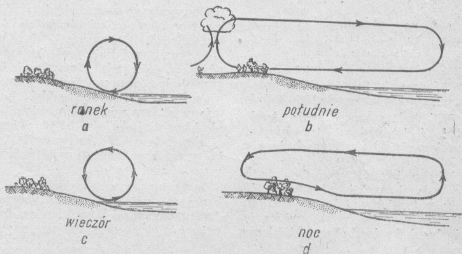
Termika wybrzeża.
