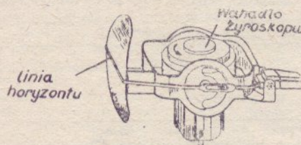
Schemat urządzenia wewnętrznego w sztucznym horyzoncie.
