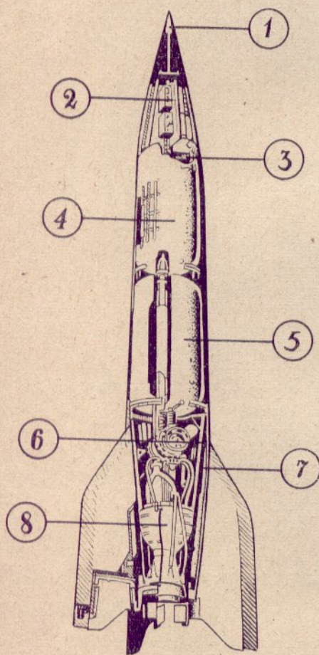
PRZĘKRÓJ RAKIETY V-2:
