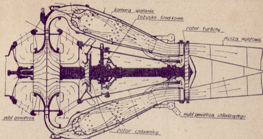
Przekrój silnika odrzutowego Rolls-Royce „Derwent V.”
