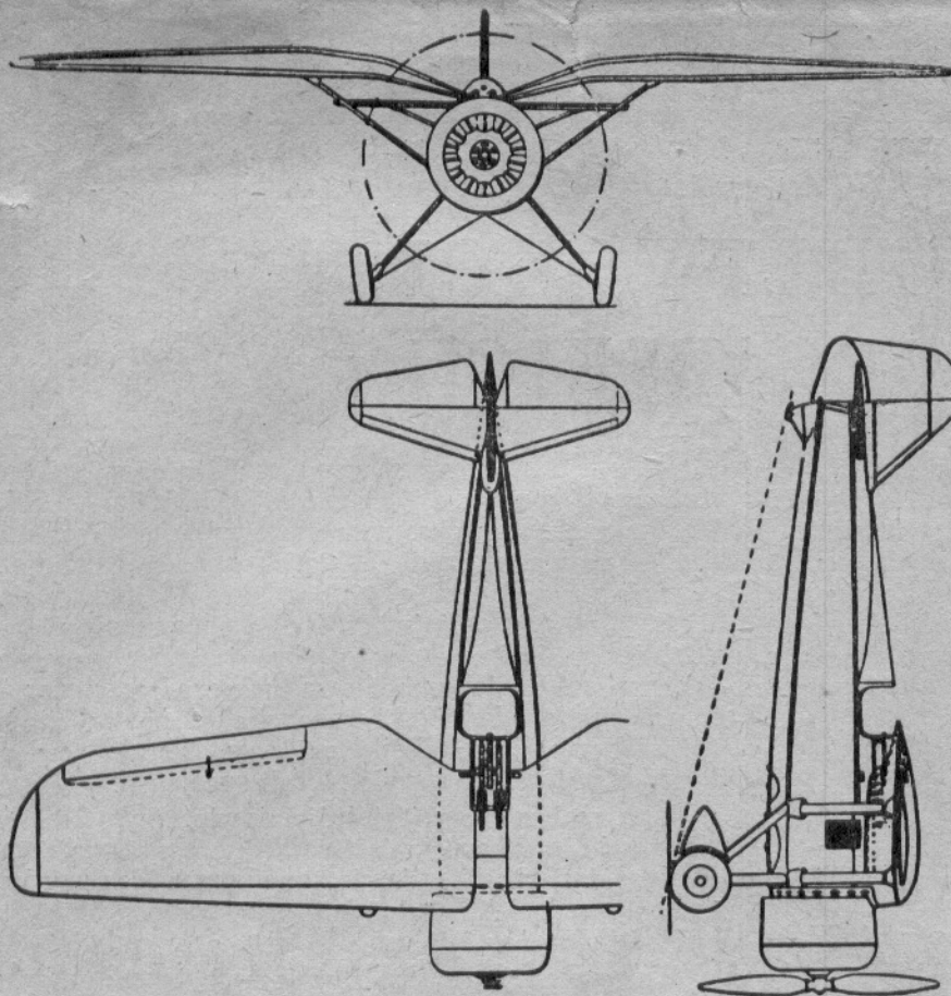
P.Z.L. P-24
