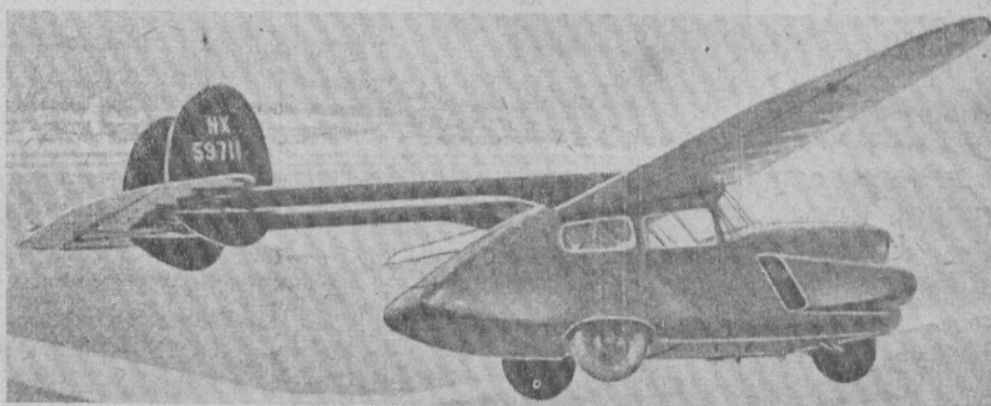
Samochód - samolot zakładów Southern Aircraft — Willis Brown „Aerocar”.
