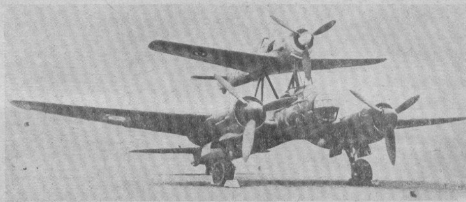
Na prawo: zespół Do-215 i FW-190.
