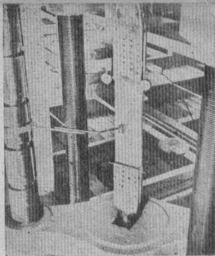
Rozrywanie nitowanej belki siłą 90 000 kg.
