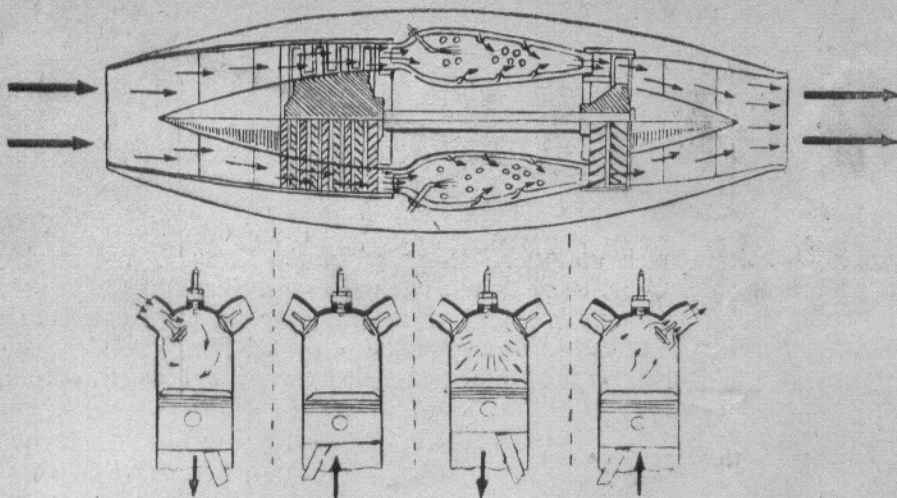
Rys. 3. 4 takty pracy silnika strumieniowo-odrzutowego i silnika tłokowego.
