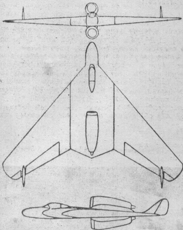
Projekt pościgowca niemieckiego P-60B o napędzie odrzutowym.
