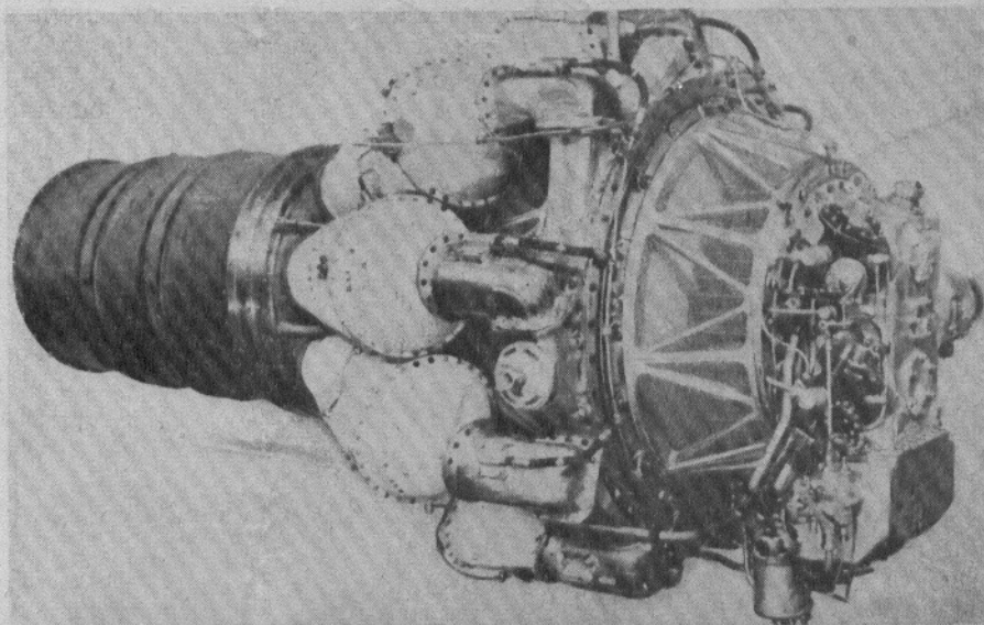
Silnik odrzutowo - strumieniowy Rolls-Royce „Nene”.
