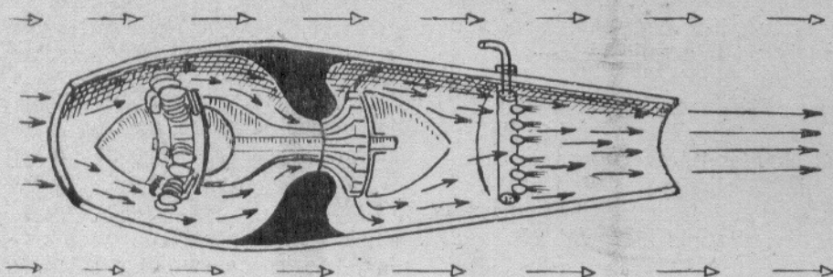
Rys. 1. Silnik strumieniowo - odrzutowy syst. Campini.
