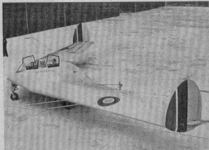
Doświadczalny szybowiec bezogonowy AW-52G
