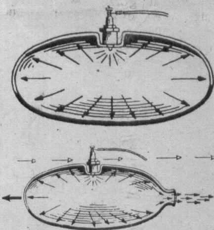
Rys. 4. Zasada działania silnika raketowego.
